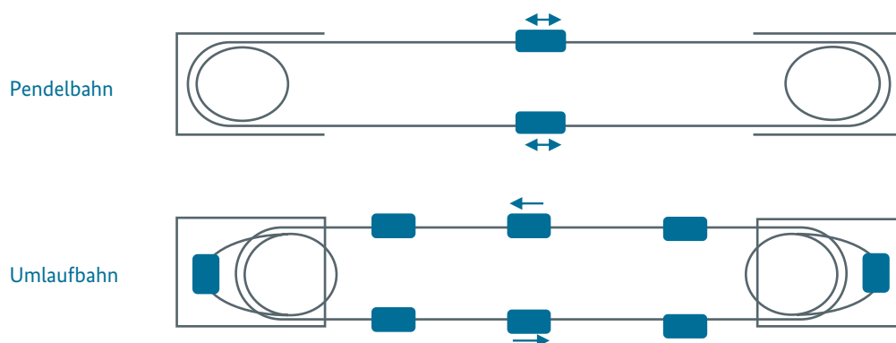
Abbildung 10: Funktionsprinzip Seilschwebbahnen
